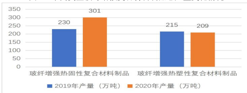
图 6、不同类型玻纤增强复合材料制品总产量变化情况
